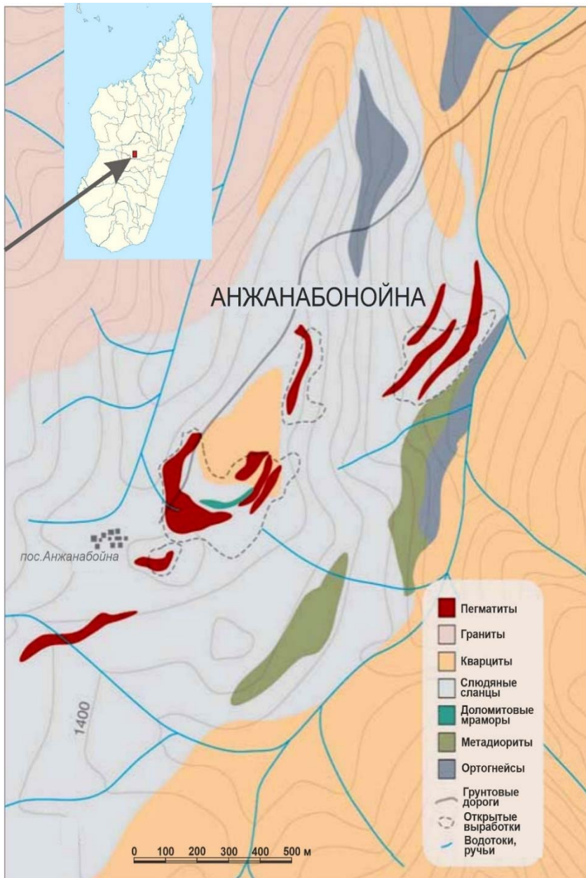
Рис. 17. Геологическая схема месторождения Анжанабойна
