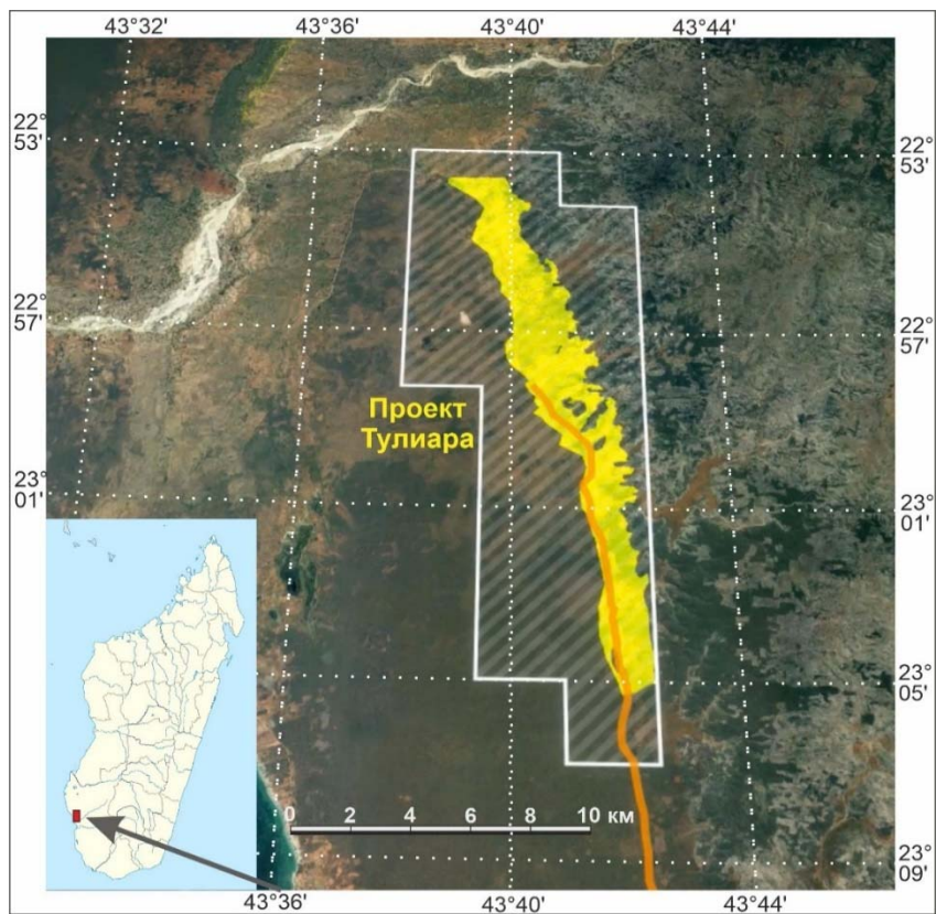
Рис. 9. Расположение дюны с пластом минерализованных песков на проекте Тулиара
