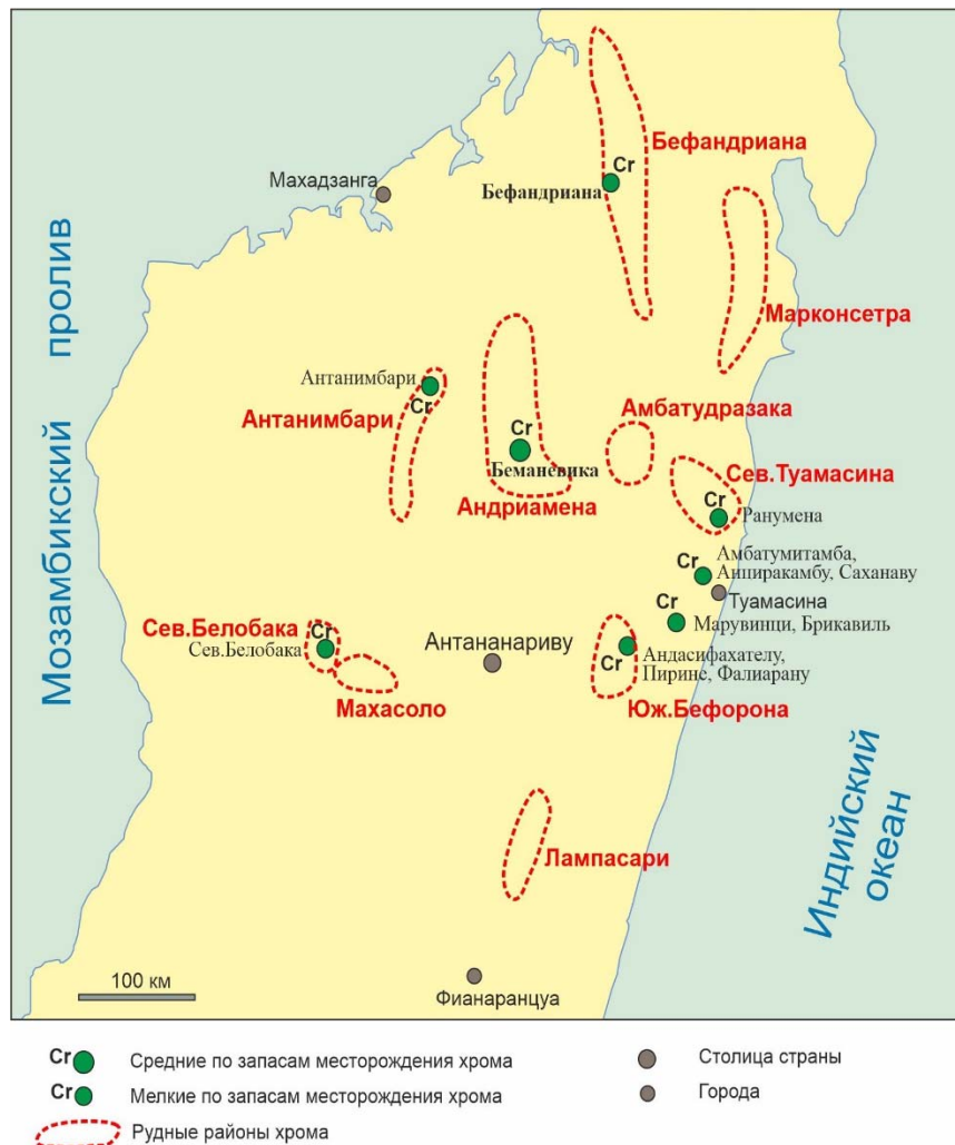
Рис. 5. Размещение основных рудных районов и месторождений хрома
