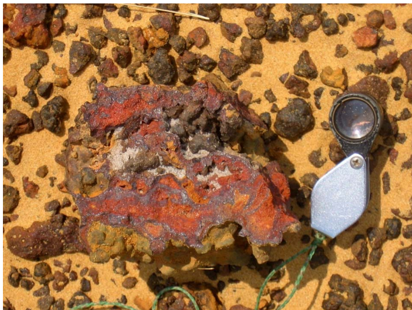
Рис. 10. Конкреция гиббсита в матрице, богатой глиной и песком на месторождении Манантенина. Размер конкреции 8×6 см
