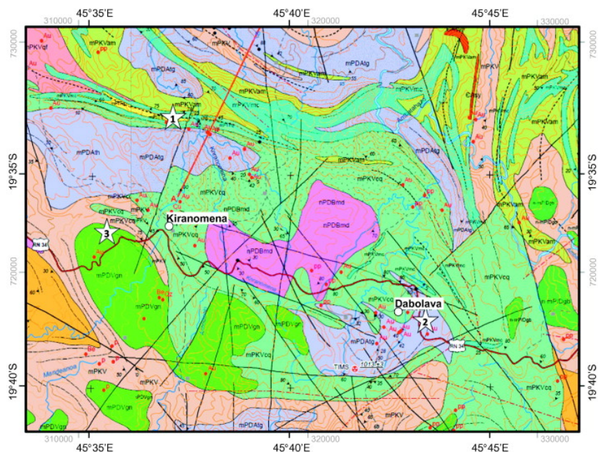
Рис. 12. Геологическая карта района золотого месторождения Даболава (Dabolava)
