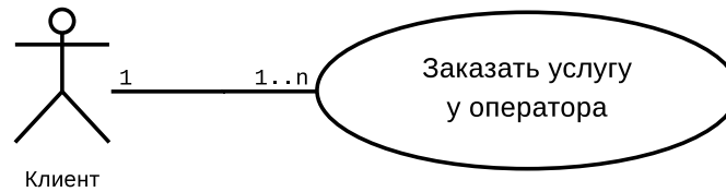
Рис. 8.4. Графическое изображение ассоциации в языке UML между актёром и вариантом использования с указанием кратности
