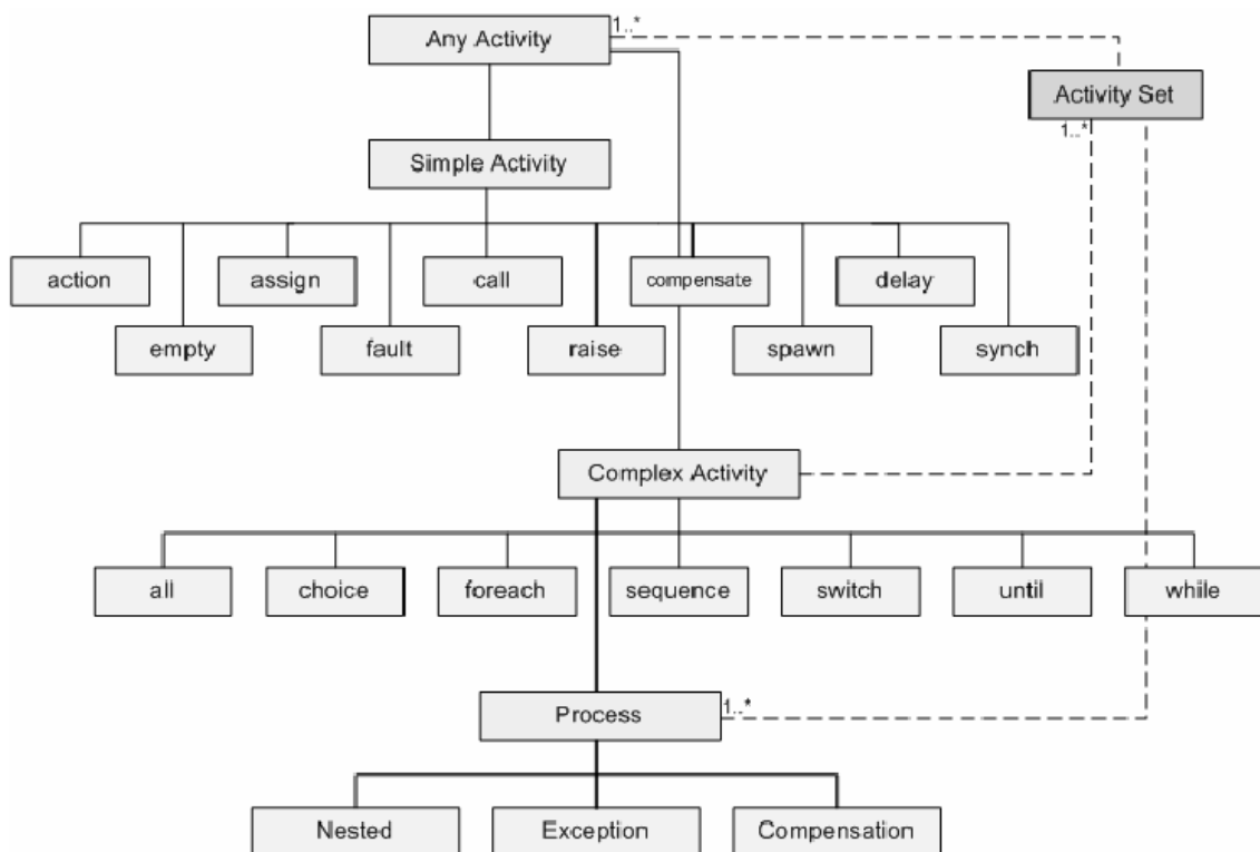
Рис. 5. Типы «действий» в BPML спецификации
