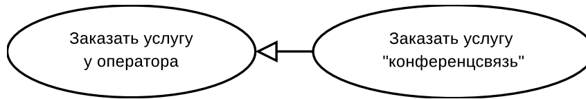
Рис. 8.7. Графическое изображение отношения обобщения в языке UML
