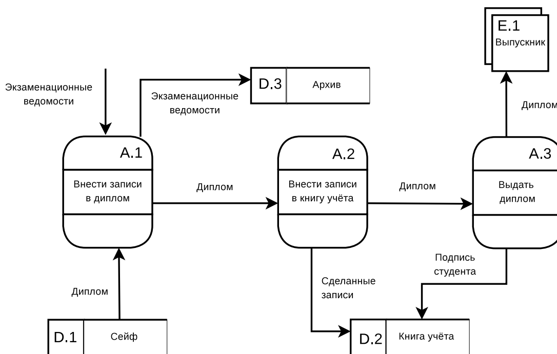
Рис. 7.4. DFD-схема «Выдача диплома»
