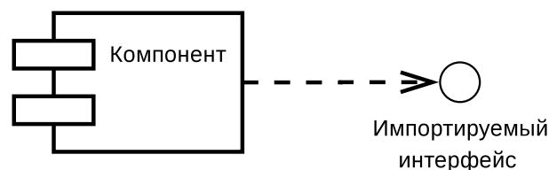
Рис. 8.34. Графическое изображение отношения зависимости на диаграмме компонентов в языке UML
