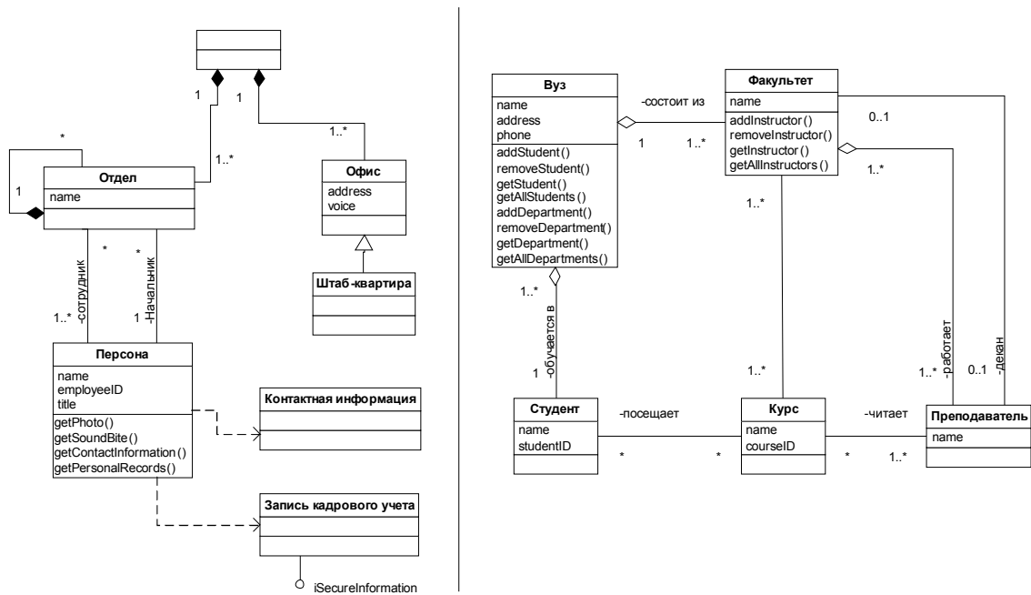
Рис. 2.Пример диаграммы классов UML
