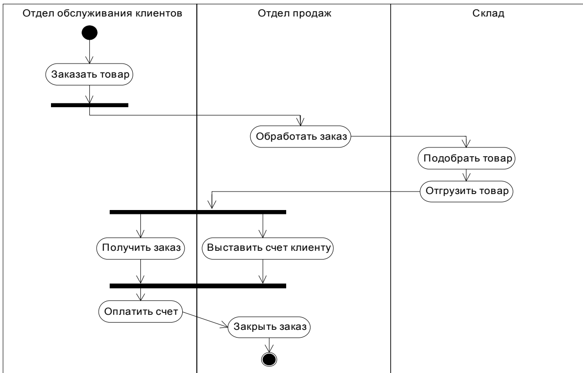
Рис. 3. Пример диаграммы деятельности UML
