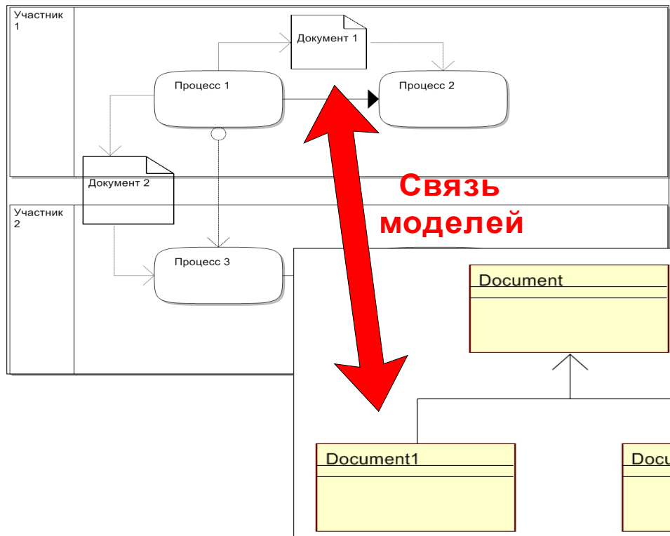
Рис. 4. Связь модели бизнес-процессов BPMN и информационной модели UML
