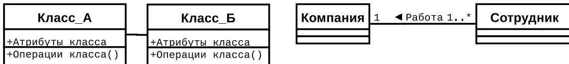
Рис. 8.11. Графическое изображение отношения ассоциации на диаграмме классов в языке UML
