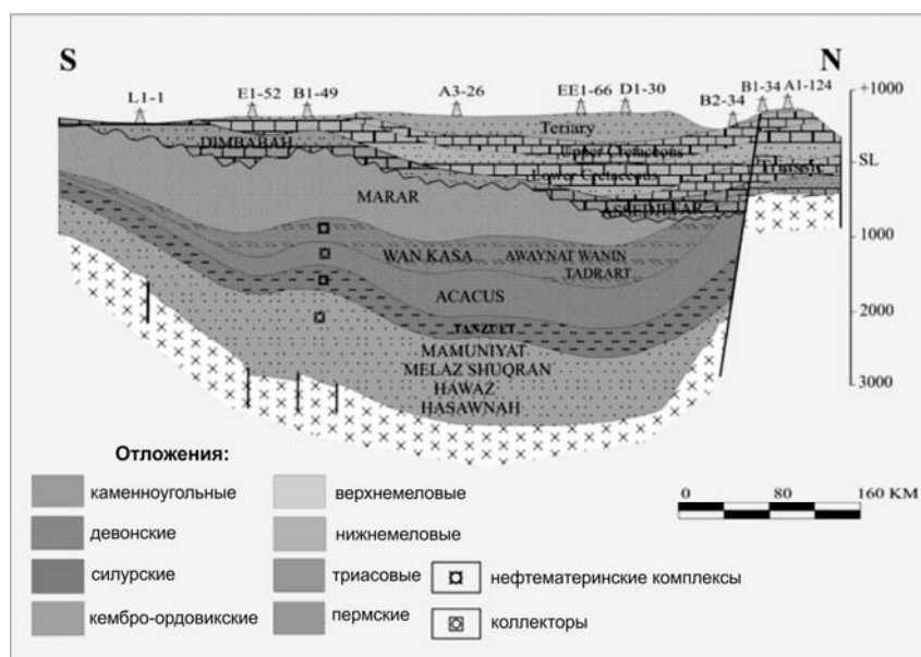
Рис. 8. Разрез с севера на юг бассейна Беркин, на территории Ливии – бассейна Гадамес (Ghadamis) (Modified after Pallas, 1980)
