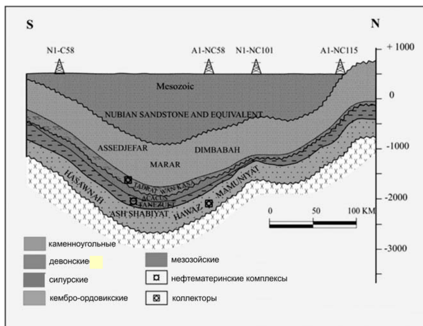
Рис. 7. Разрез с севера на юг бассейна Иллизи, на территории Ливии – бассейна Мурзук (Murzuq) (Modified after Pallas, 1980)
