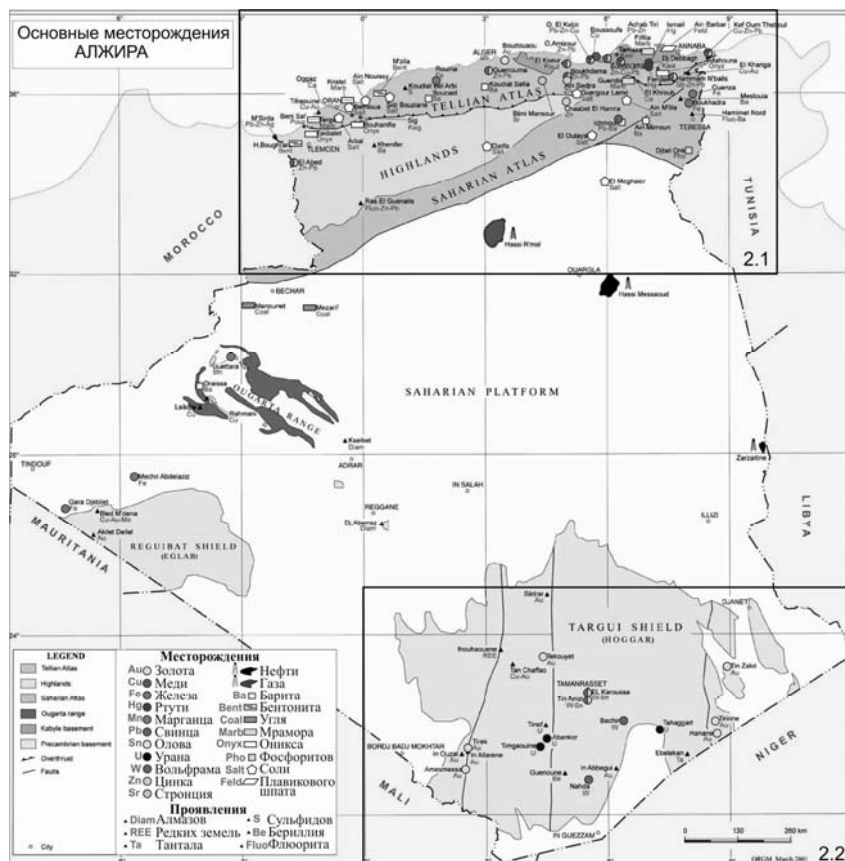
Рис. 2. Схема размещения основных месторождений и проявлений Алжира
