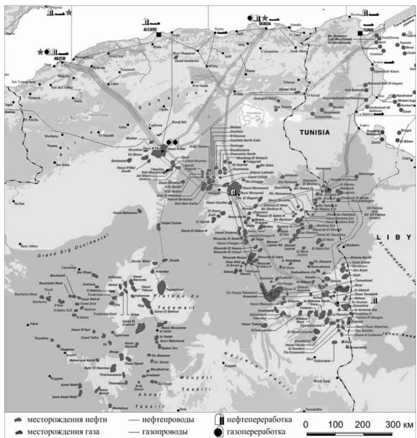
Рис. 6. Месторождения нефти и газа Алжира
