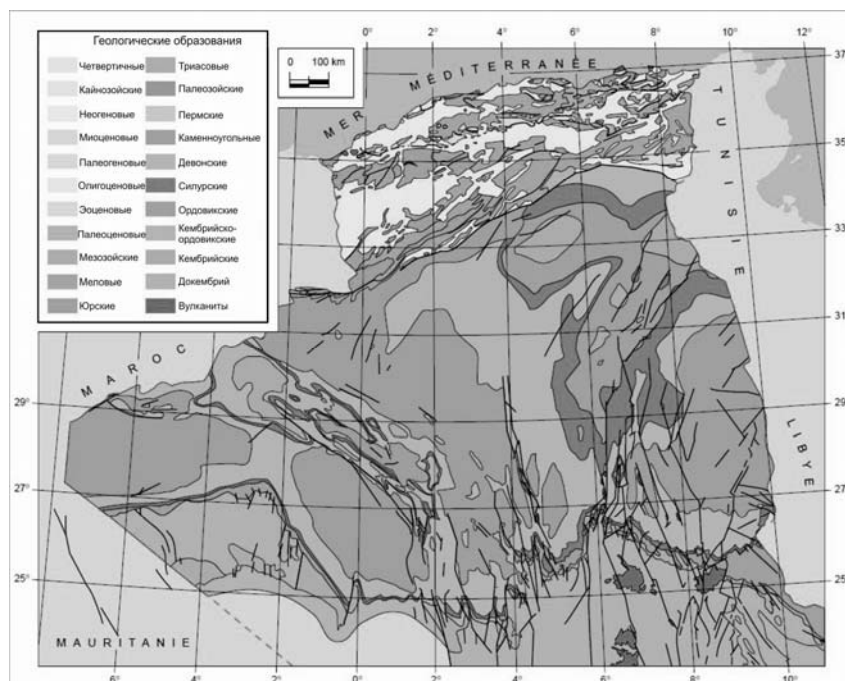
Рис. 1. Геологическая карта основной части Алжира
