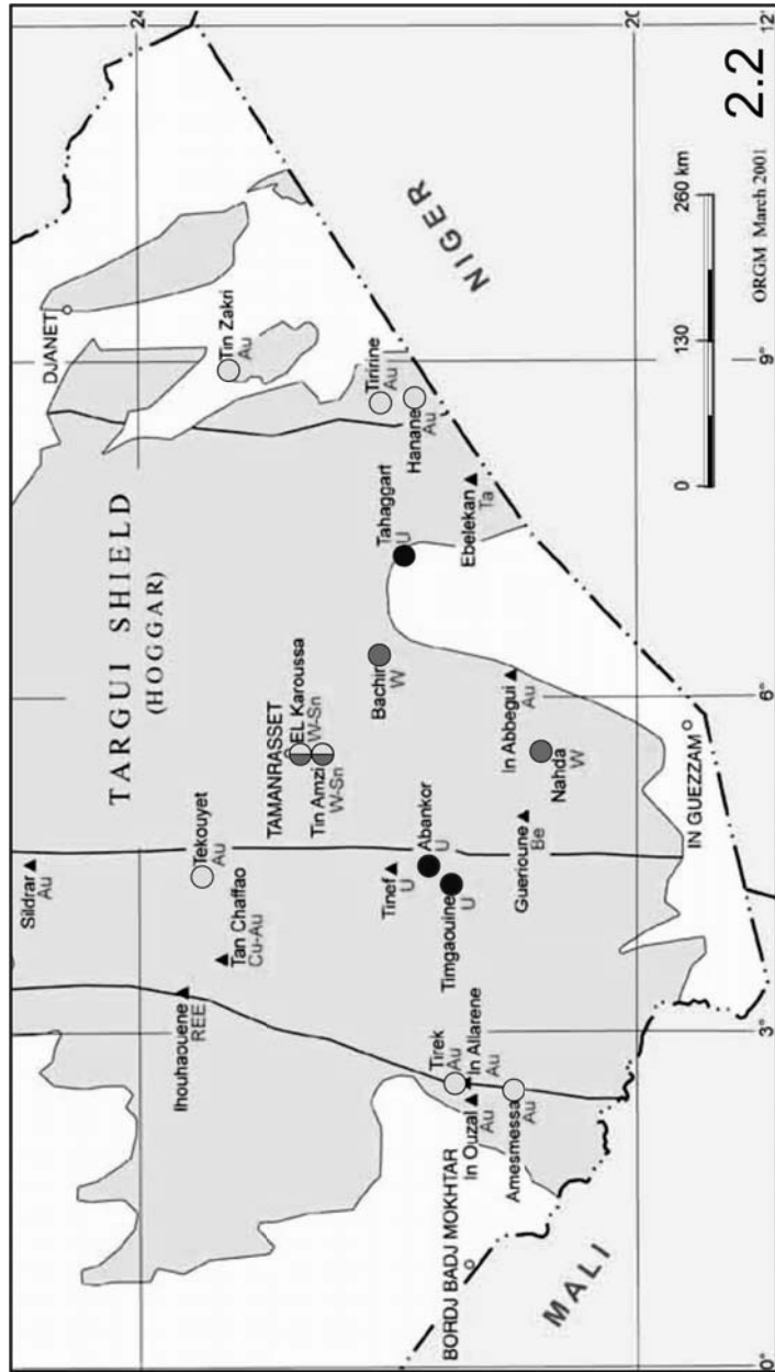
Рис. 3. Схема размещения основных месторождений и проявлений Юга Алжира Условные обозначения приведены на рис. 2
