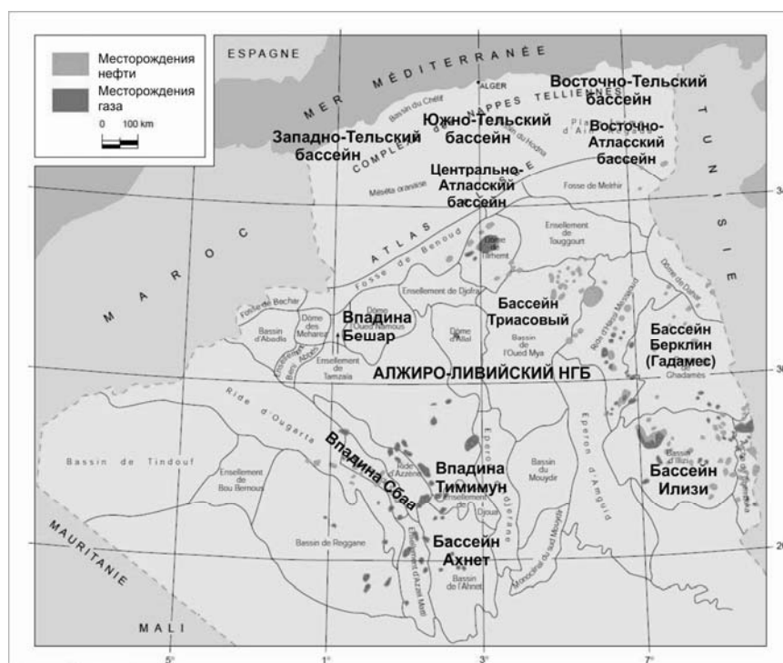
Рис. 5. Схема нефтегазоносности Алжира
