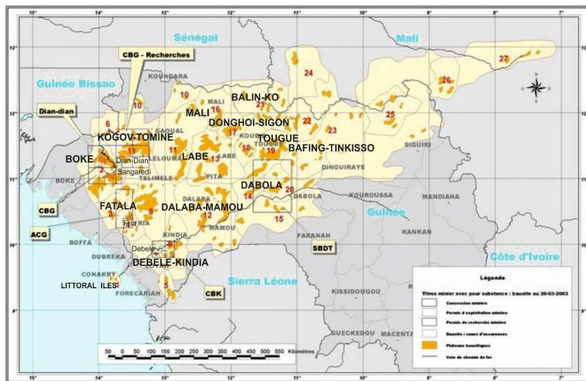
Рис. 5. Расположение основных бокситоносных районов Гвинеи (районы выделены оранжевым цветом )
