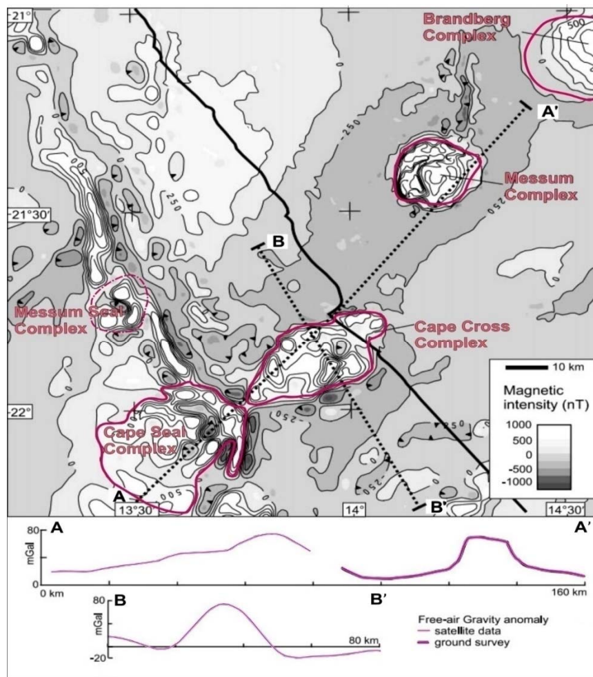
Рис. 5. Карта интенсивности магнитного поля и гравиметрические аномалии интрузивных комплексов площади Кейп-Кросс
