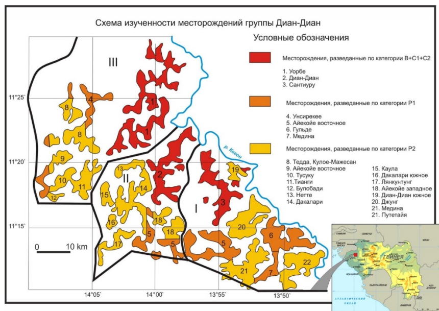
Рис. 7. Месторождения группы Диан-Диан в бокситоносном районе Боке
