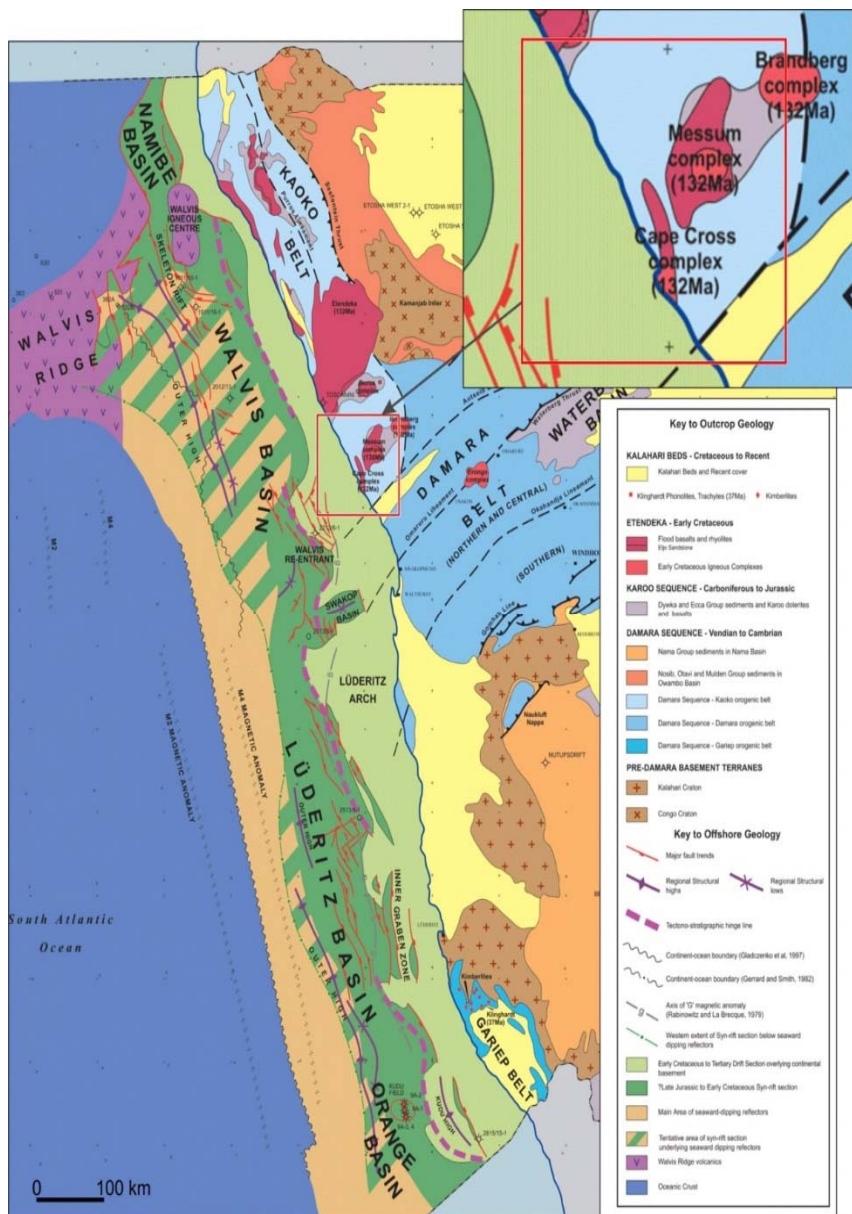
Рис. 3. Структурно-геологическая карта Намибии с увеличенным фрагментом изучаемой площади Кейп-Кросс
