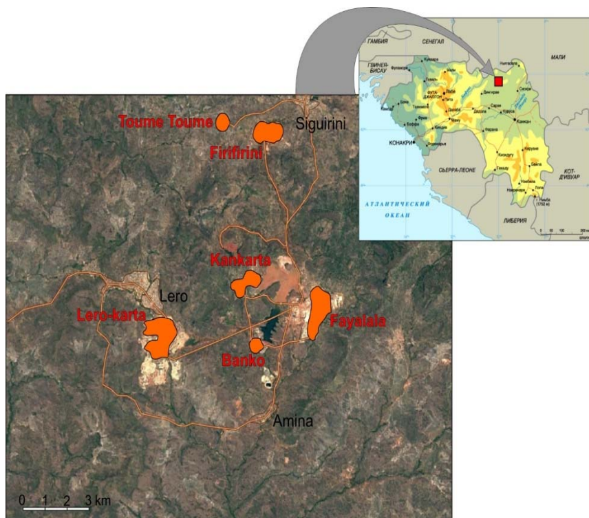
Рис. 9. Расположение основных рудников (их названия даны красным цветом) на золоторудном объекте Лефа (Lefa) компании Nordgold
