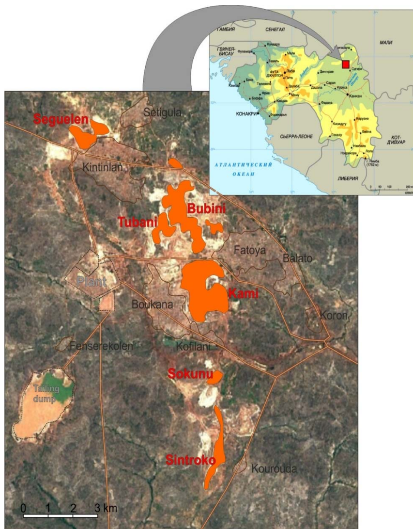
Рис. 11. Расположение основных рудников (их названия даны красным цветом ) на золоторудном объекте Сигуири (Siguiro) компании Ashanti Company of Guinea
