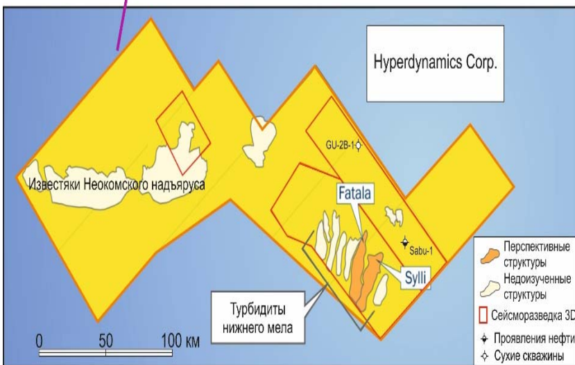
Рис. 2. Блоки глубокого шельфа, изученные работами Hyperdynamics Corp
