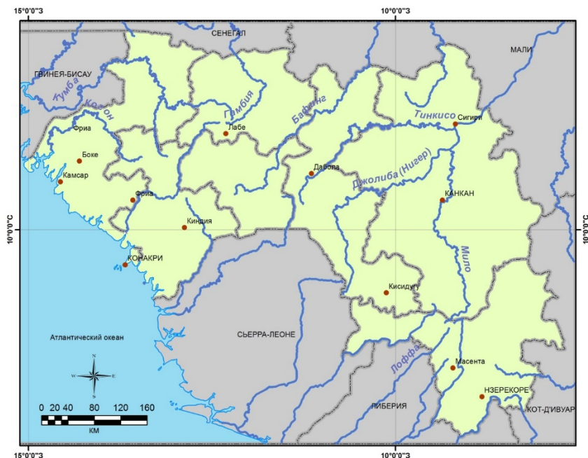
Рис. 13. Гидрологическая карта Гвинеи
