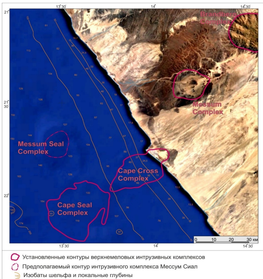
Рис. 4. Гранитоидные комплексы Брандберг, Мессум, Кейп-Кросс, Кейп-Сял и Мессум Сял
