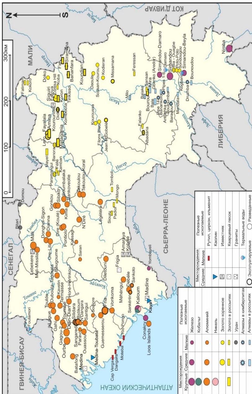
Рис. 1. Основные месторождения полезных ископаемых Гвинейской Республики
