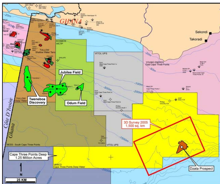
Рис. 3. Размещение выявленных месторождений нефти и газа на шельфе Ганы
