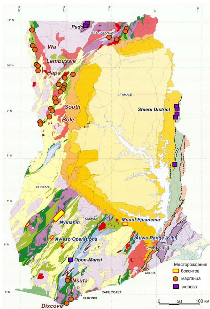
Рис. 4. Месторождения железа, марганца и бокситов
