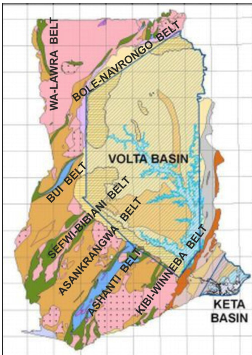
Рис. 5. Золоторудные пояса Ганы
