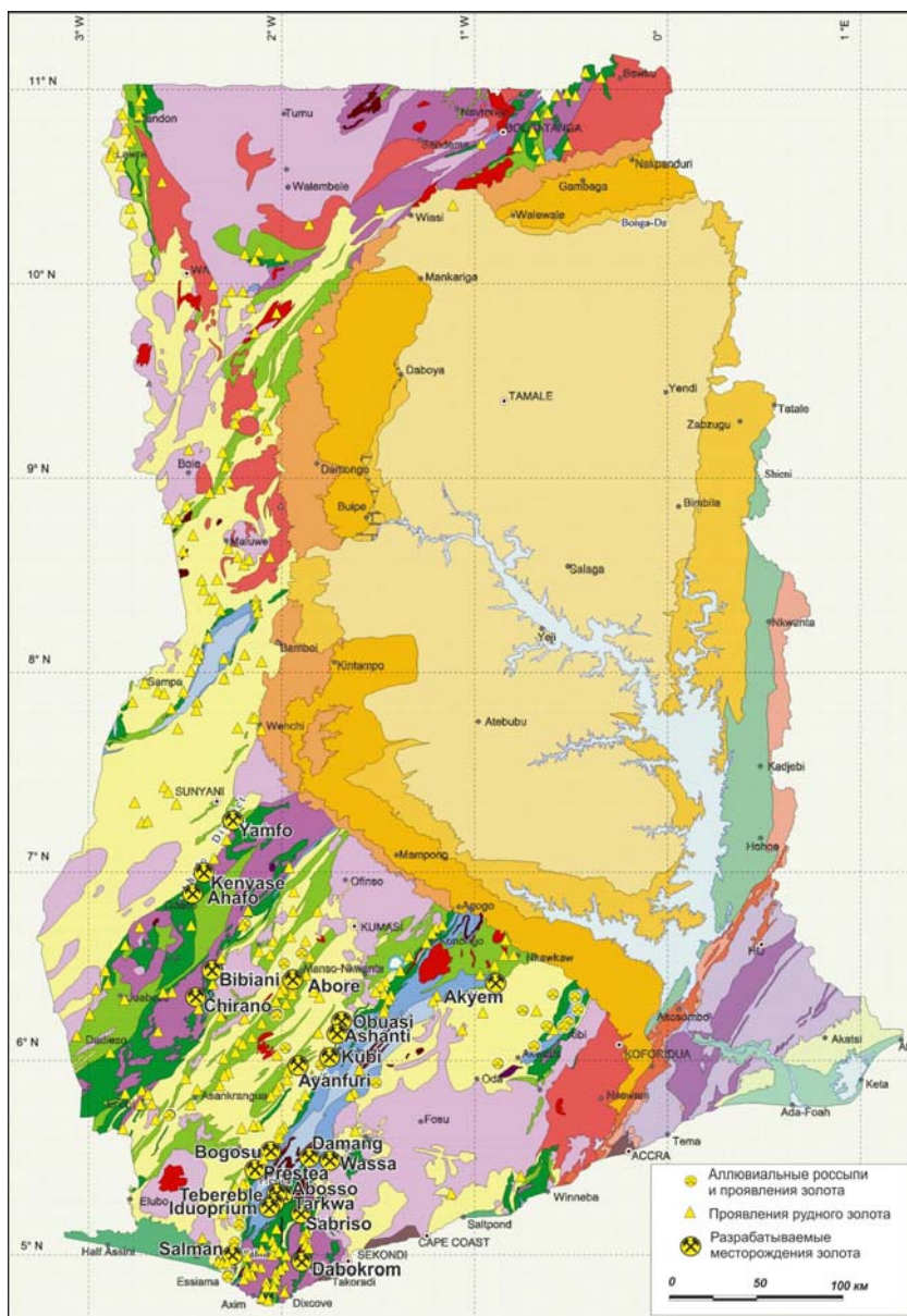
Рис. 6. Золотые коренные и россыпные месторождения золота, их проявления
