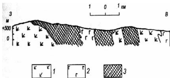
Рис. 2.6. Схематический разрез открытых Гусевогорского и Качканарского месторождений (по В.В. Авдониному и др.) ваннадиеносных титаномагнетитов. 1-амфиболиты, 2-габбро, 3-рудные залежи
