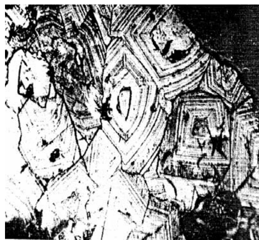
Рис. 2.4. Структура идиоморфнозернистая агрегата повеллита \text{Ca}(\text{MoO}_4) . Увеличение 40 раз. Аншлиф. Месторождение Каджаран, Армения. (По М.П. Исаенко)
