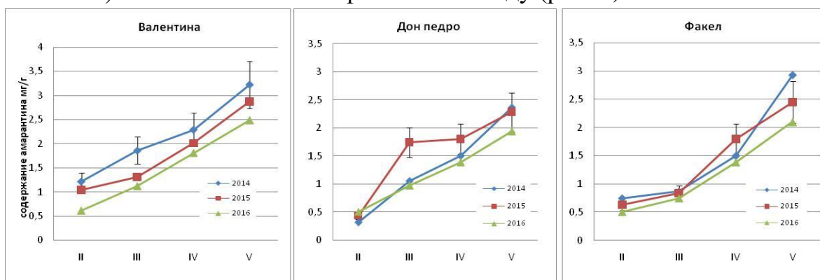
Рис. 4. Содержание амарантина (мг/г) в соцветиях сортов амаранта в зависимости от фазы онтогенеза в разные годы исследований (2014-2016 годы)
