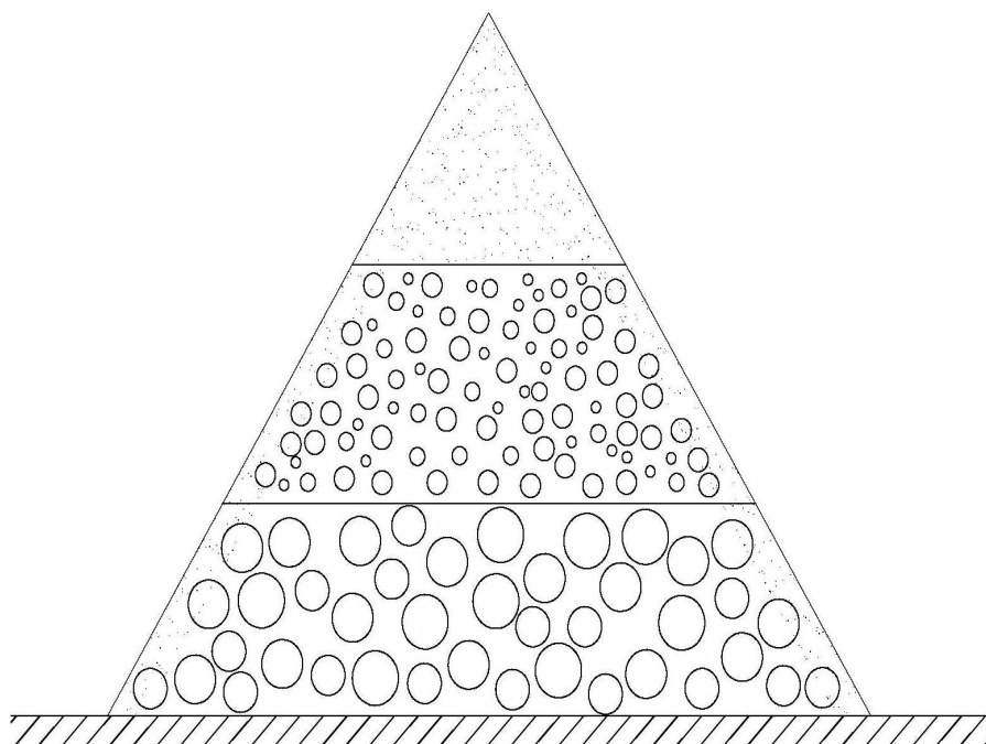
Рис. 4. Структура террикона по гранулометрическому составу.
